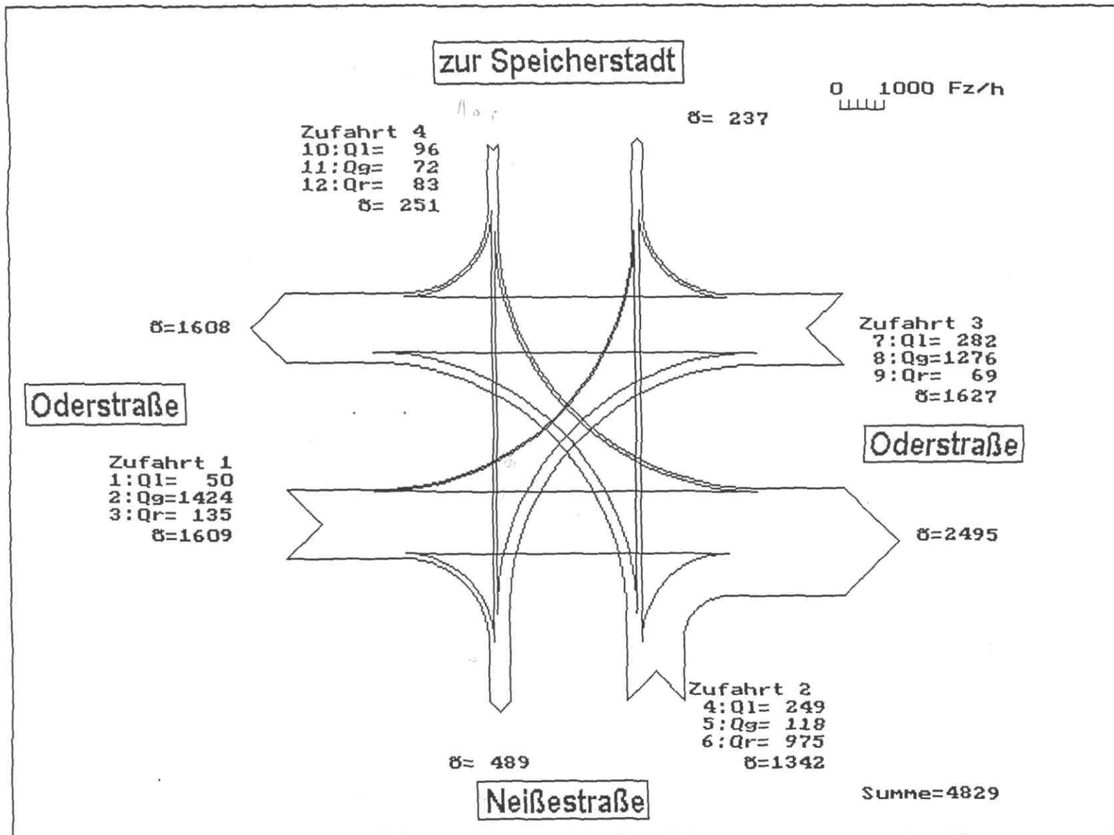
Plan 13.4: Knotenstrombelastungsplan Oderstraße/ Neißestraße (Angaben in Kfz/ 4 Stunden)
