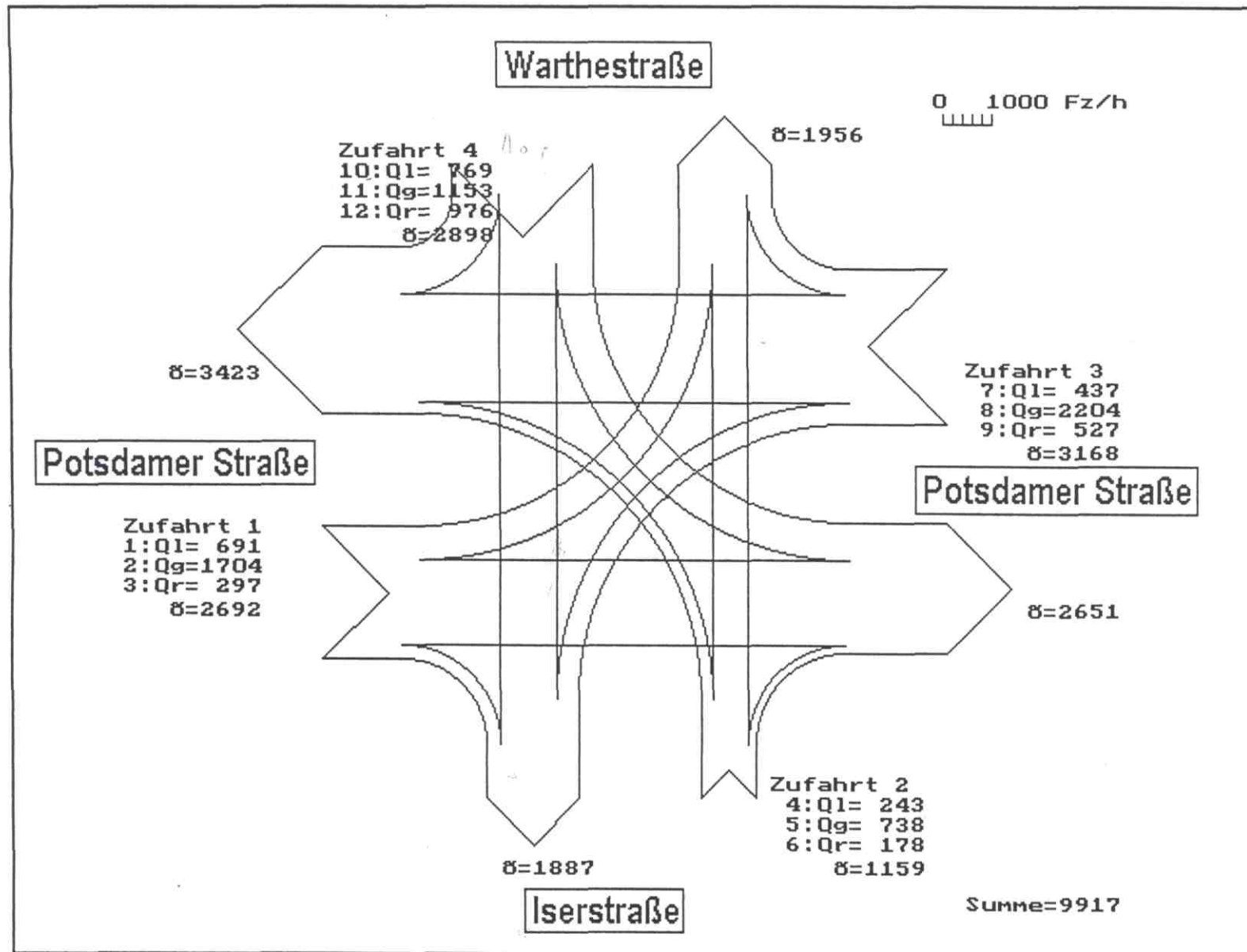
Plan 13.3: Knotenstrombelastungsplan Liebigplatz (Angaben in Kfz/ 4 Stunden)
